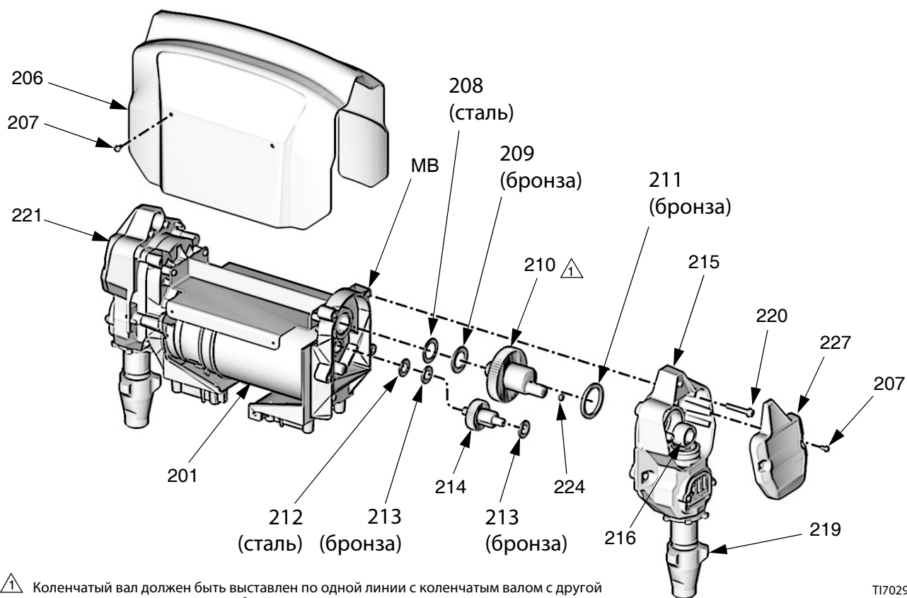
Рис.14. Корпус привода
